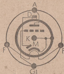
Sockelschaltung
